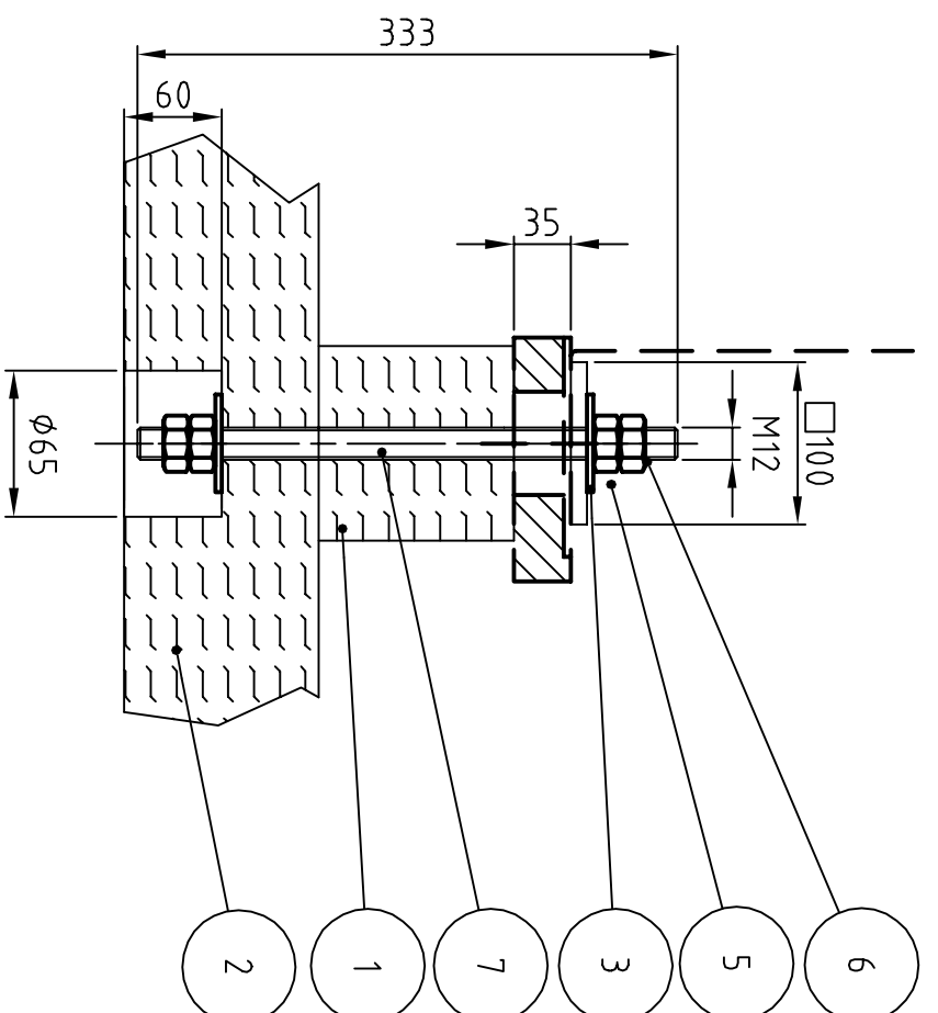
A-A (1:5)
